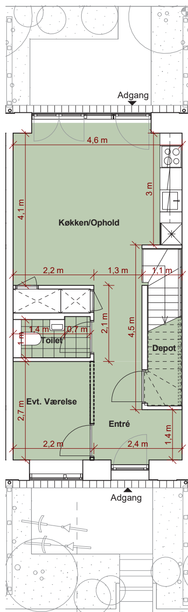
Stue etage
